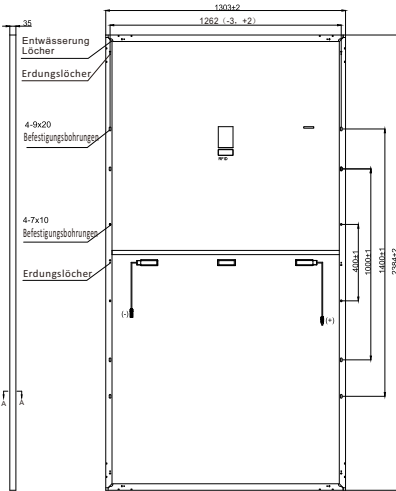
Abmessungen des PV-Moduls
