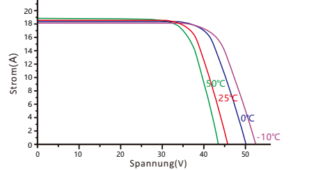
IV-Kennlinien bei verschiedenen Temperaturen (AM1.5, 1000W/m 2 )
