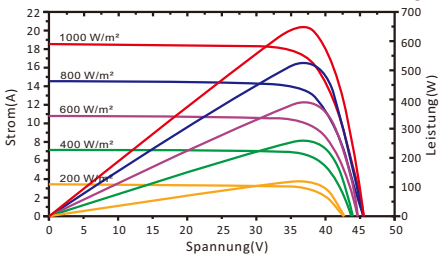
RSM132-8-655M I-V-Kennlinien bei unterschiedlichen Einstrahlungen
